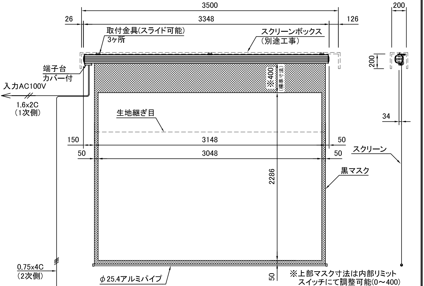
外観図 S=1/30
