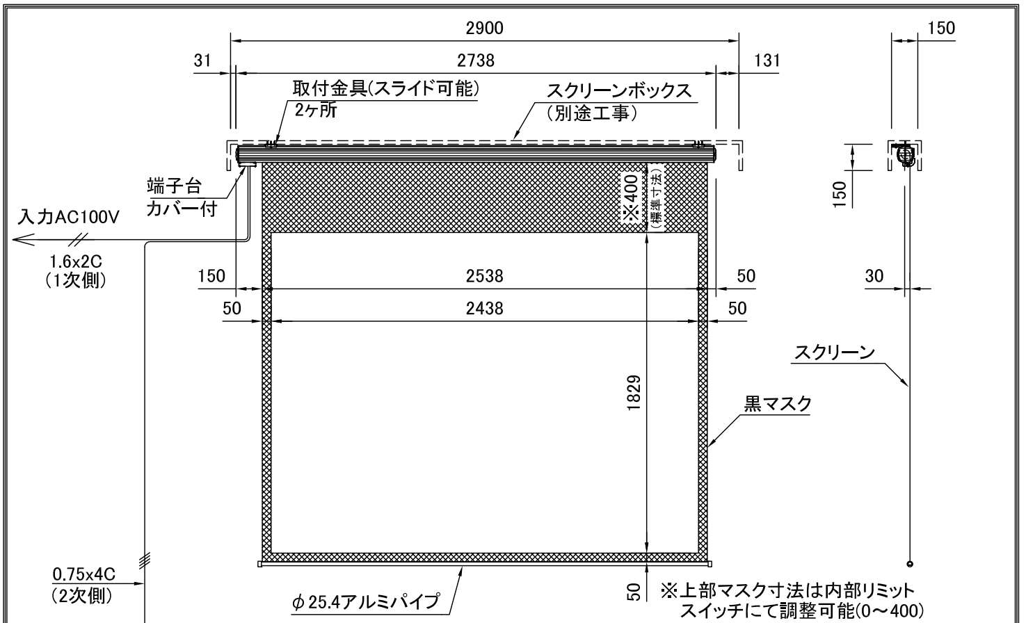
外観図 S=1/30
