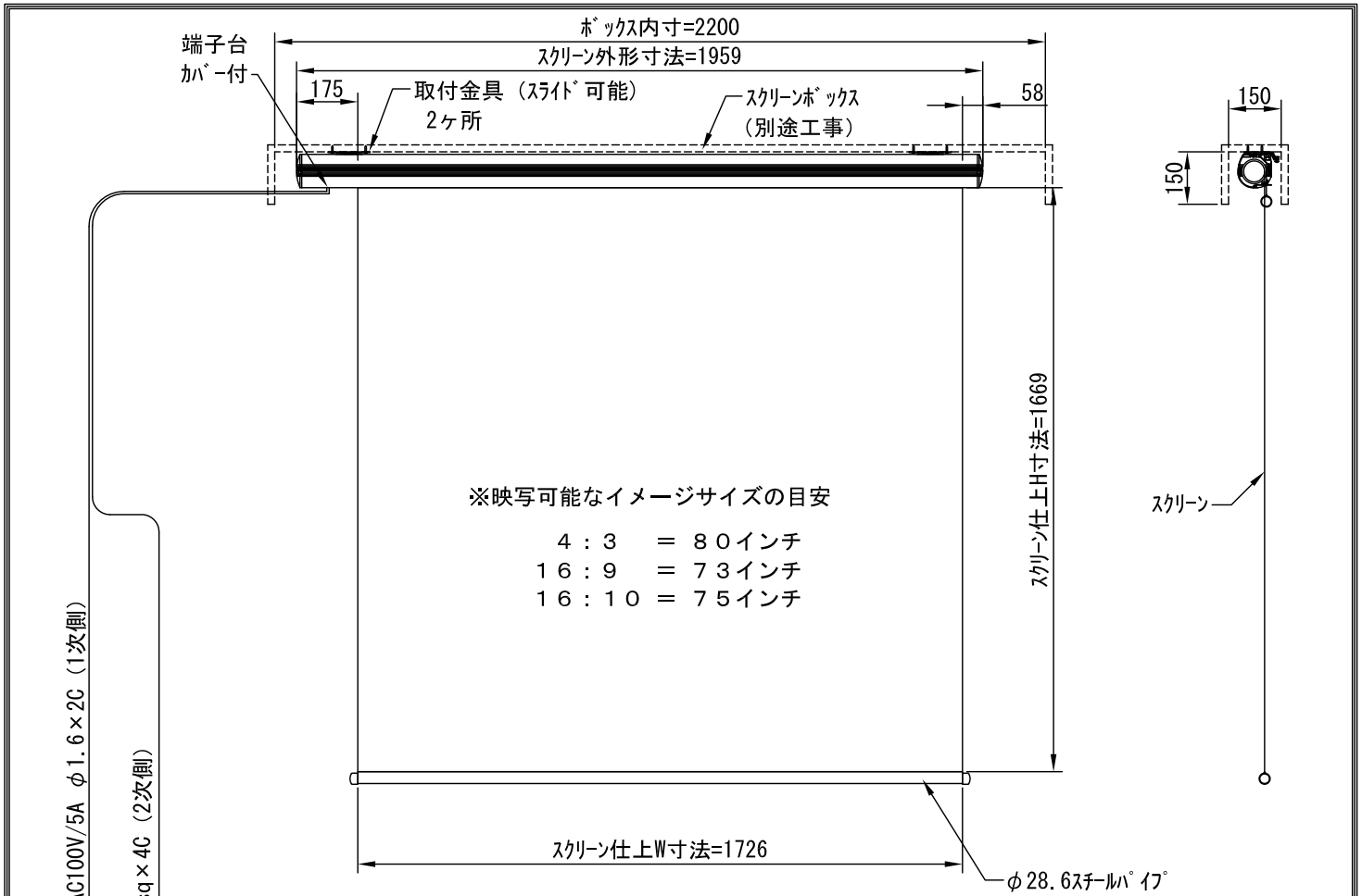
外觀図 1/20
