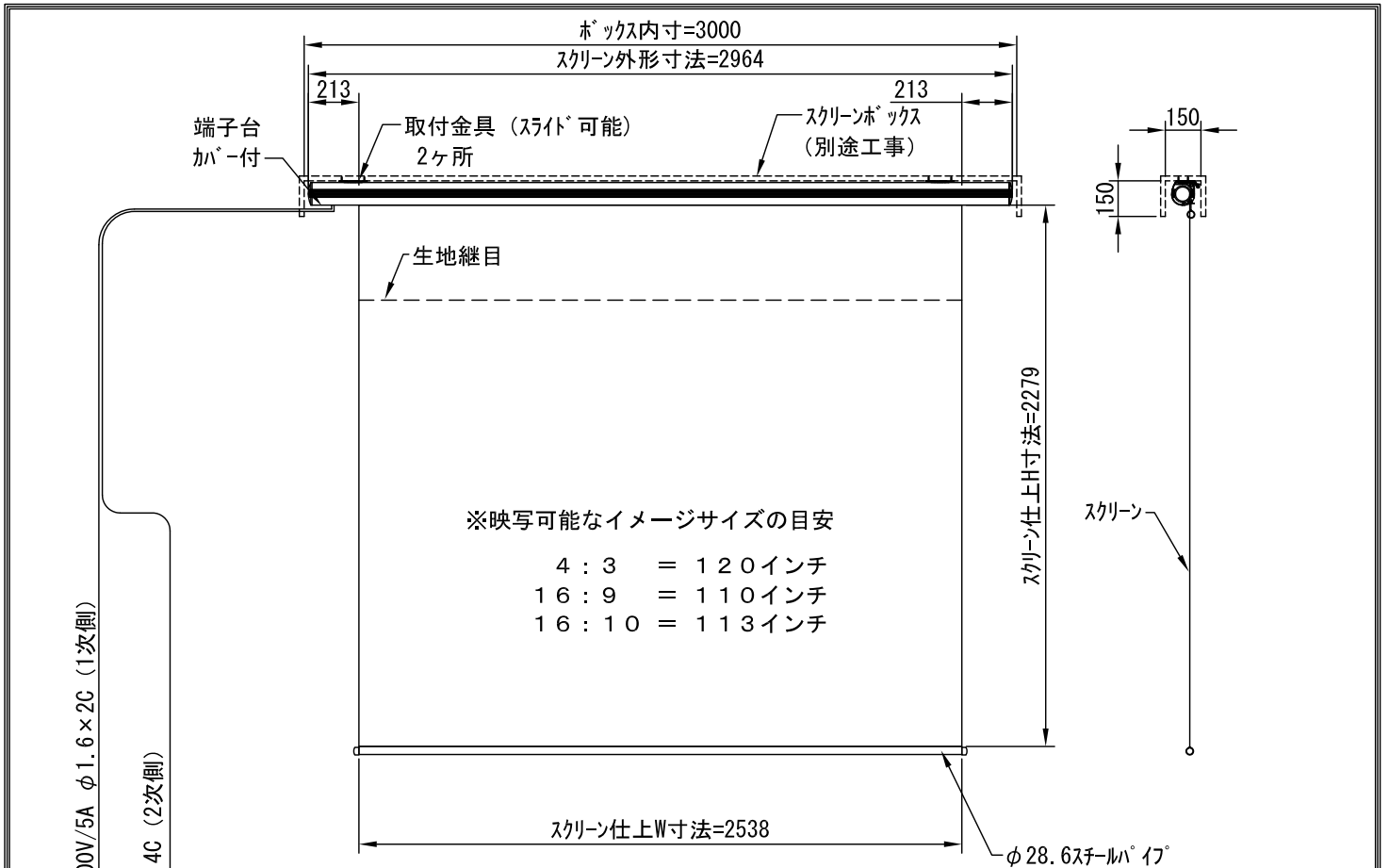
外観図 1/30
