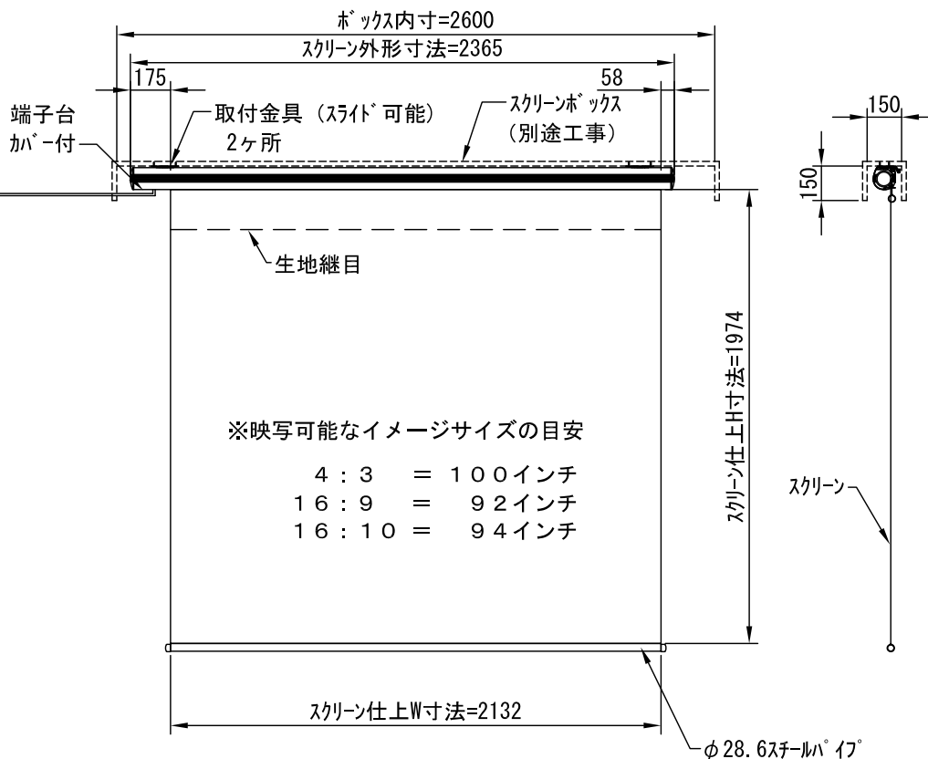
外觀図 1/30
