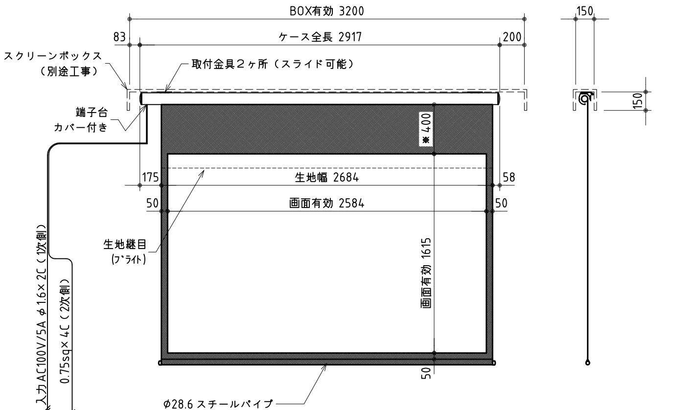
外觀図 S=1/30
