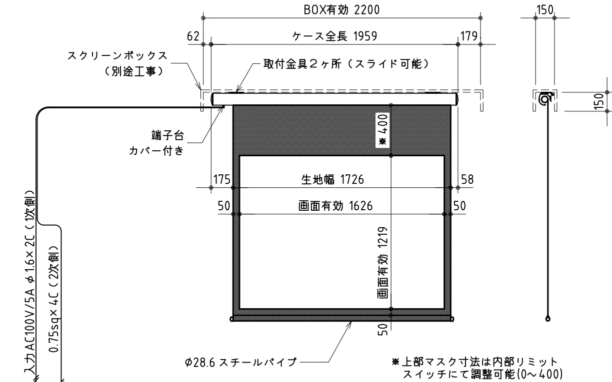
外觀図 S=1/30
